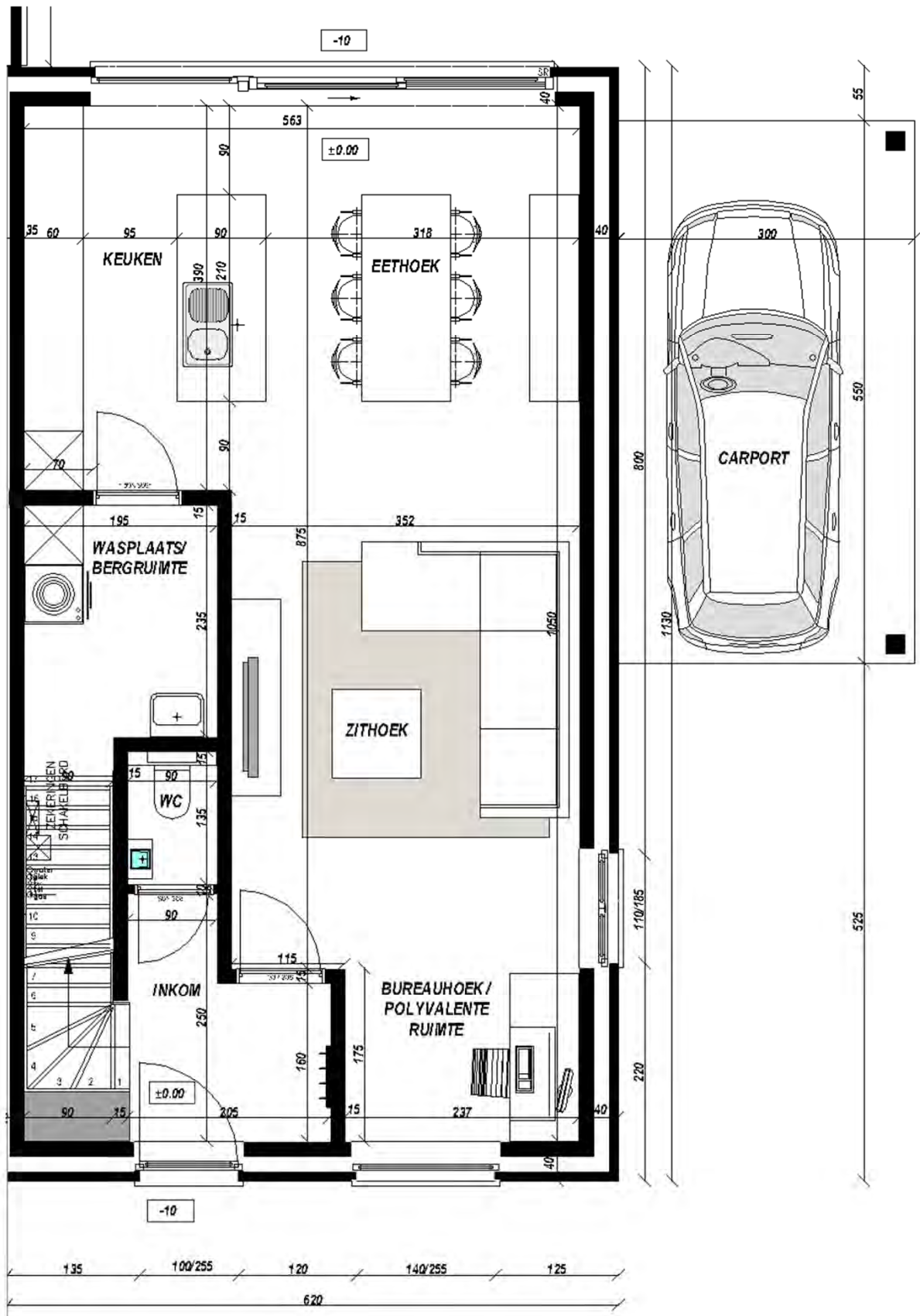
LOT 4 GELIJKVLOERS 1 opp. : 70,12 m 2
